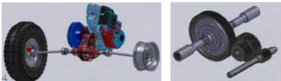
Figura 15. Ensamble y subensamble de Sistema de Transmision.
