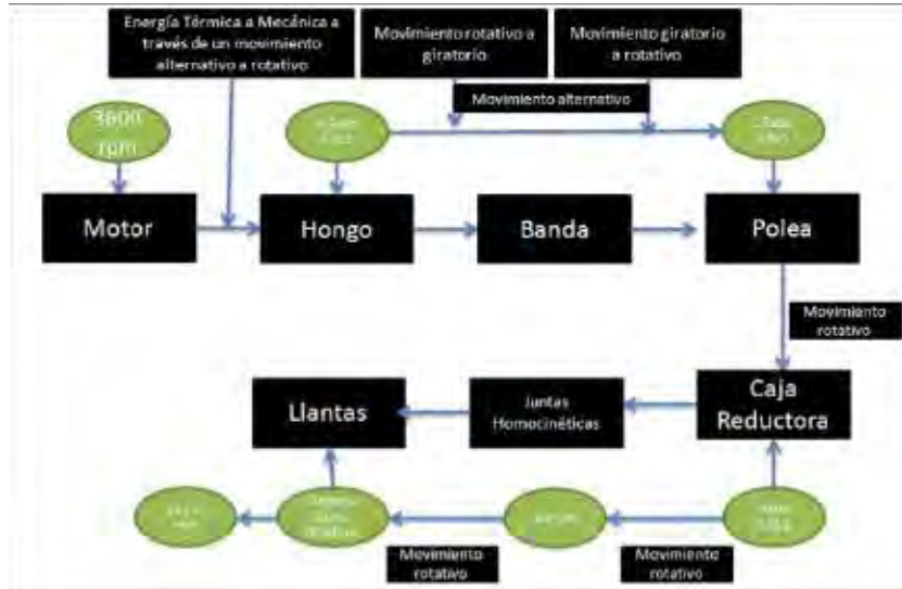
Figura 12. Diagrama del análisis de movimiento en el sistema de la Transmisión.
