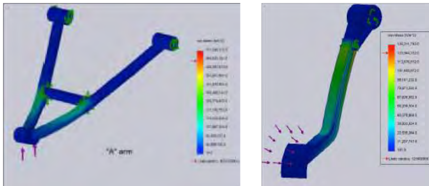
Figura 14. Analisis de Esfuerzo de la horquilla en la suspension delantera y pedal de freno.
