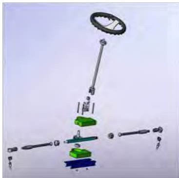
Figura 9. Modelado CAD Direccion.
