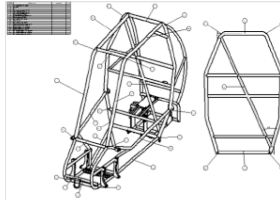
Figura 16. Elementos que componen la jaula antivuelco.
