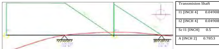
Figura 13. Analisis momento flexionante y cortante de la flecha
